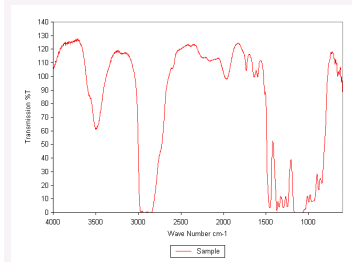
Infrarot-Spektrum
