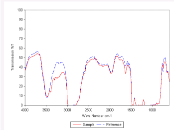
Infrarot-Spektrum
